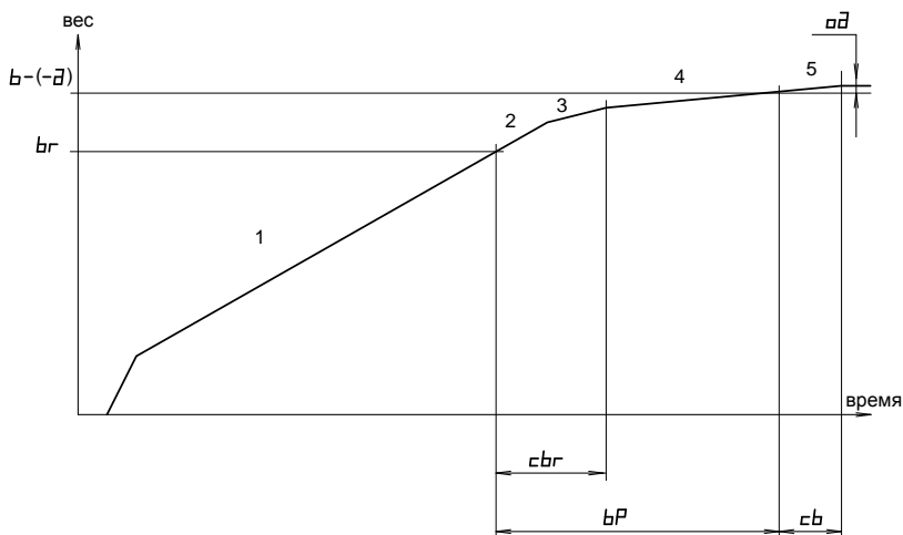
Рис. 1а. Диаграмма дозирования.
