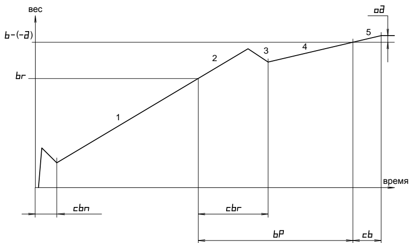
Рис. 1б. Диаграмма дозирования под давлением.
