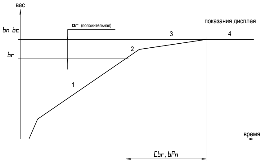
Рис. 2а. Диаграмма грубого дозирования.
